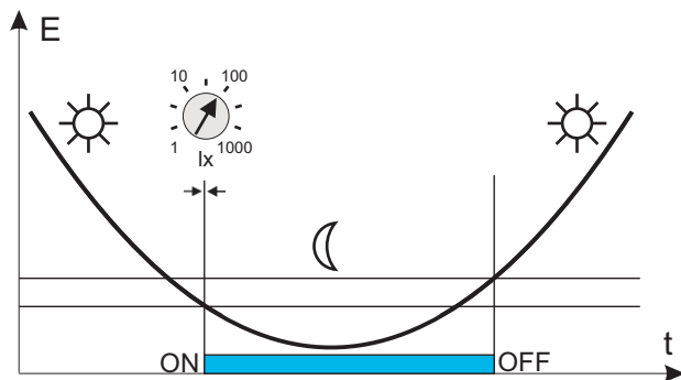
Abb. 3.: Schema des Wirkungsbereichs des Dämmerungsschalters TS-52-3
