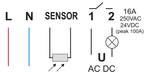
Abb. 4: Anschlusspläne des DÄMMERUNGSSCHALTERS TS-51-2 wenn der Empfänger mit einer anderen Spannung als 230V AC betrieben wird. Die maximalen Spannungen U sind: 250V DC und 24V AC.
