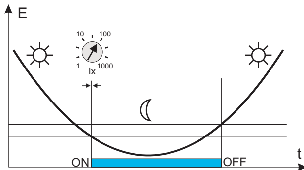
Abb. 5: Schema des Wirkungsbereichs des Dämmerungsschalters TS-51-2
