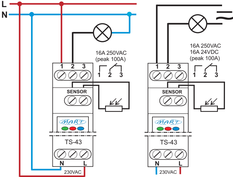
Bild 2: Anschlusschema des DÄMMERUNGSSCHALTERS TS-43-4
