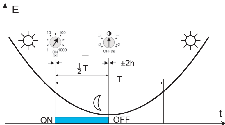
Bild 3: Funktionsschema des DÄMMERUNGSSCHALTERS TS-43-2
