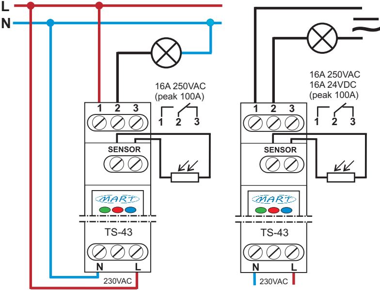
Bild 2: Anschlussschema des DÄMMERUNGSSCHALTERS TS-43-2
