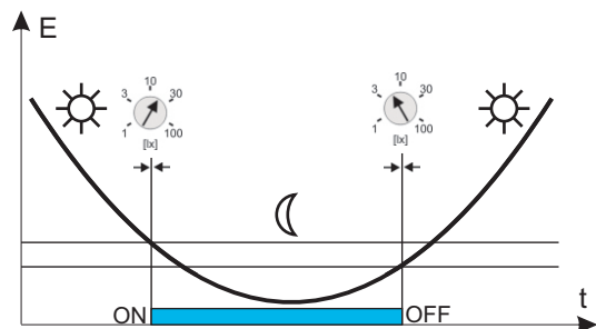
Bild 3: Funktionsschema des DÄMMERUNGSSCHALTERS TS-42-4
