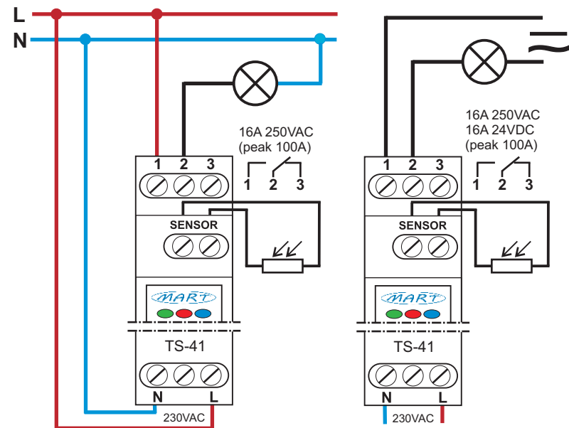
Bild 2: Anschlussschema des Dämmerungsschalters TS-41-4
