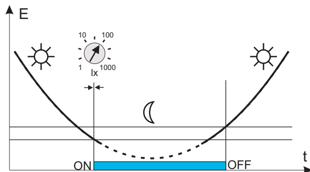
Bild 3: Schema des Wirkungsereichs des Dämmerungsschalters TS-41-3.4
