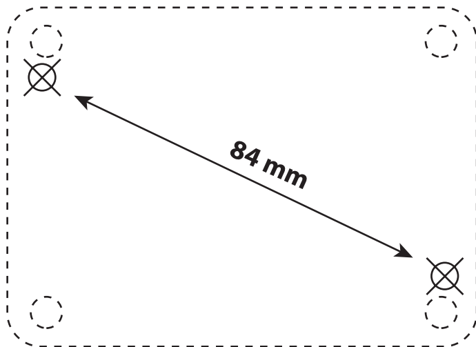
Bild 2.: Schablone für Bohrlöcher zur Befestigung des Dämmerungsschalters TS-31-2
