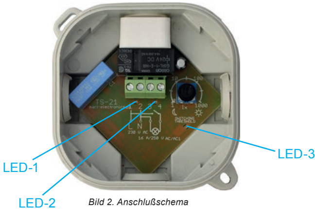
Bild 2. Anschlussschema
