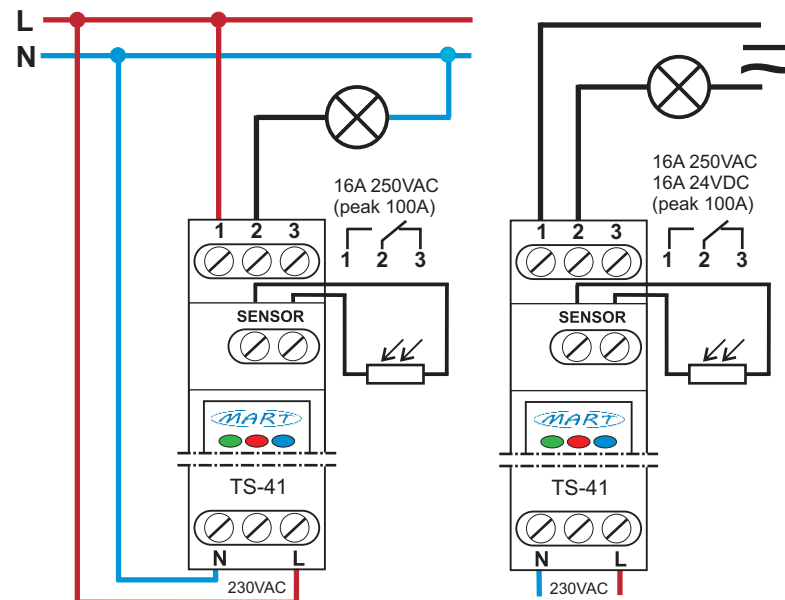
Rys. 2.: Schematy podłączenia AUTOMATU ZMIERZCHOWEGO TS-41-2.
